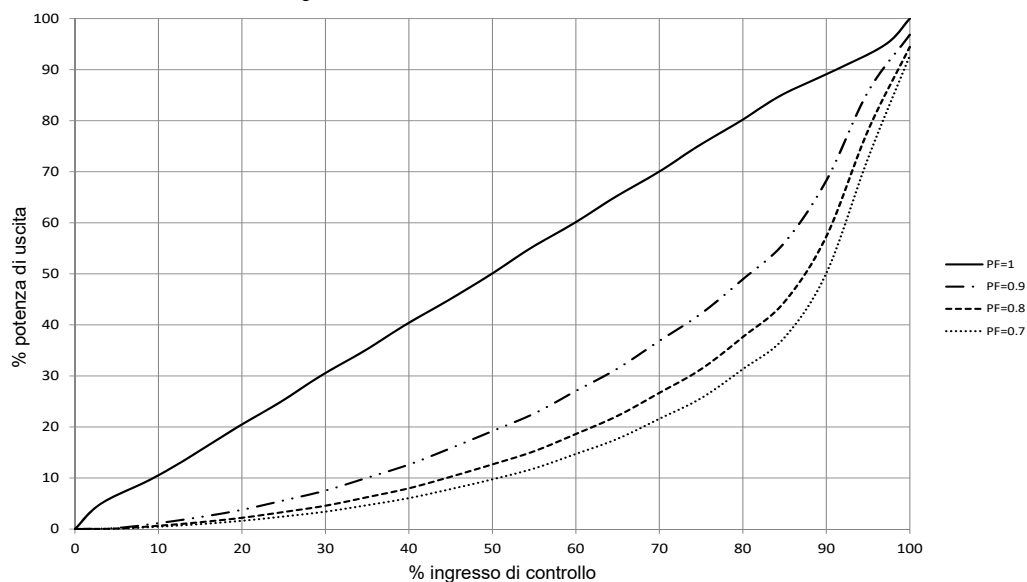
Modalità 1: commutazione angolo di fase
