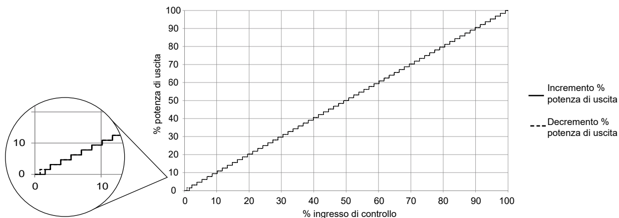
Modalità 2: 1x commutazione ciclo completo
