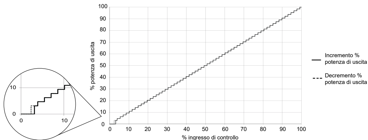
Modalità 3: 4x commutazione ciclo completo
