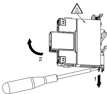
Smontaggio da guida DIN
