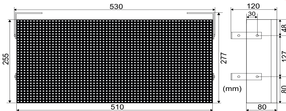
Fig. 3 Dimensions DISCRSE
