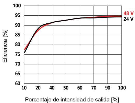
Eficiencia frente a carga de salida (230 VCA)
