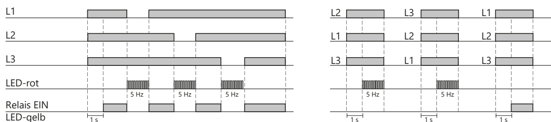
Fig. 1 Vollständiger Phasenausfall, Phasenfolge
