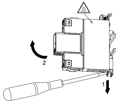
Demontering fra DIN-skinne
