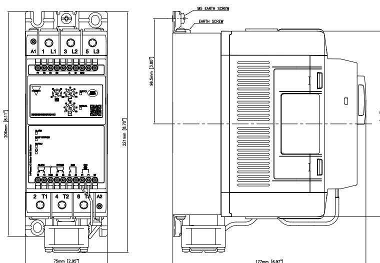
Fig. 4 RSGD..100..VX311C (tavlemonteret)
