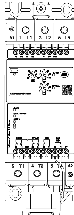
Fig. 6 RSGD 75 mm
